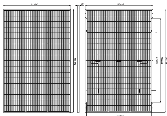
Todas las dimensiones están en mm. El dibujo de arriba es una representación gráfica del producto.
